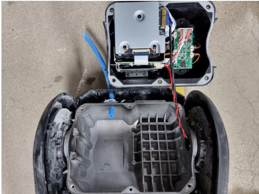
< 사진3. IP6X 시험 후 내부 >
