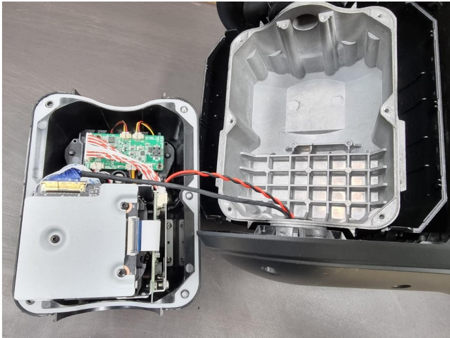
< 사진5. IPX6 시험 후 내부 >
