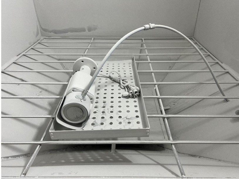
< 사진3. IP6X 시험 후 외부 >
