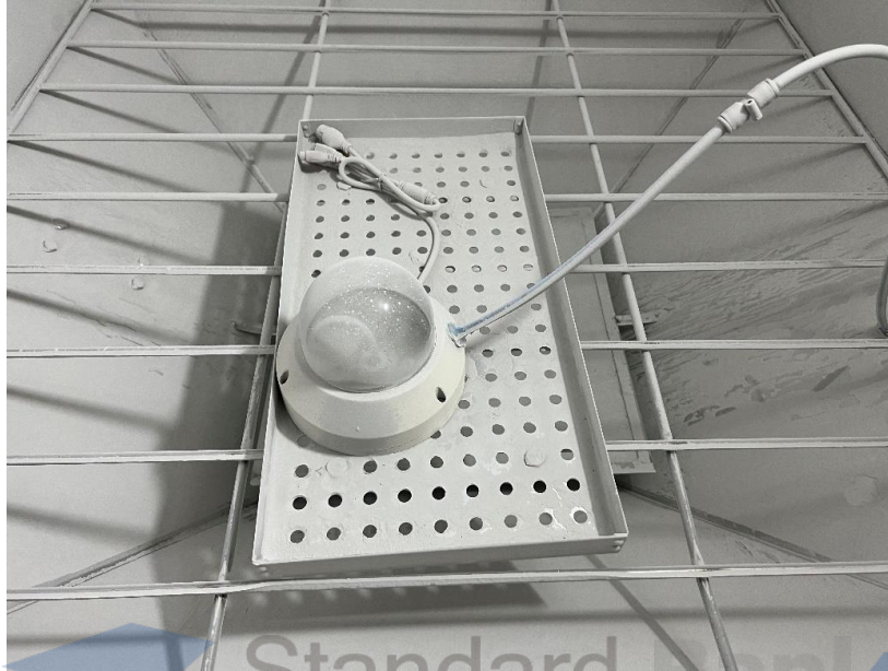
< 사진2. IP6X 시험 후 외부 >
